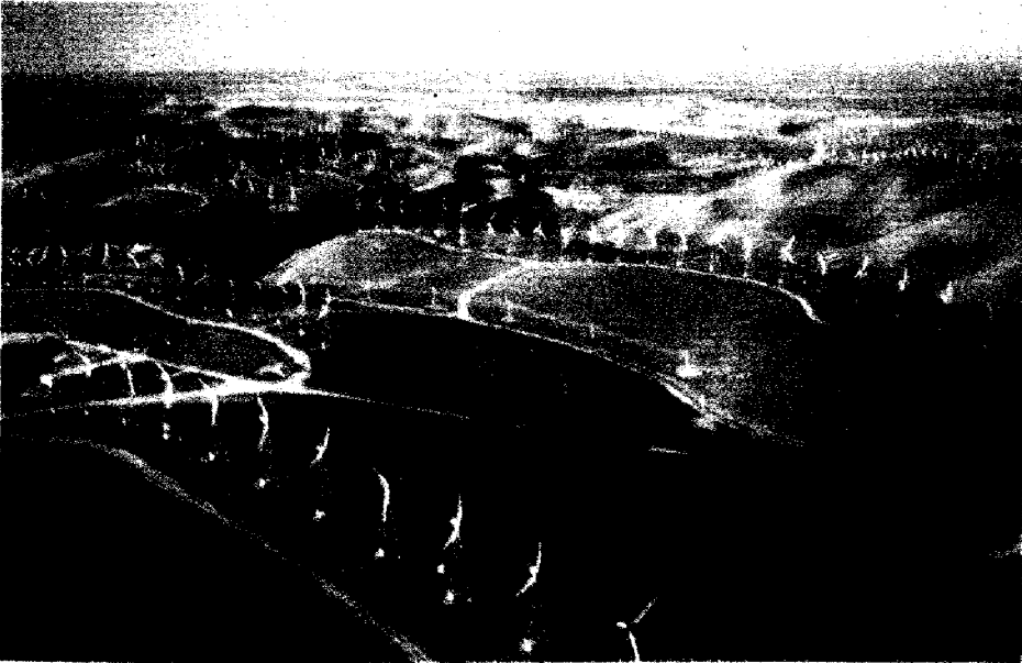
प्लेट 2. डेनमार्क का स्काई नदी का पवन ऊर्जा फार्म। इसमें वी-27-225 किलोवाट क्षमता की गति नियंत्रित 342 वेस्टास पवन टर्बाइनें लगी हैं।
